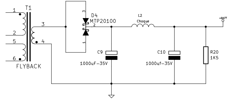
Secundário da fonte com filtro IEM
