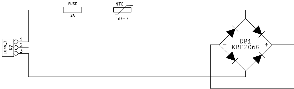
Primário da fonte sem filtro IEM
