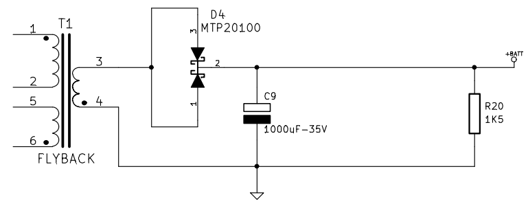
Secundário da fonte sem filtro IEM
